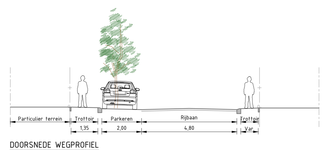
DOORSNEDEN WEGPROFIEL Schaal 1:100
